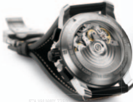
ETA VALJOUX 7750
